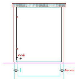
Pohľad D
