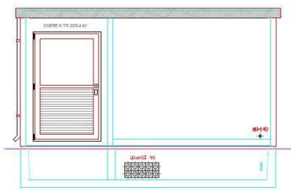
Pohľad A
