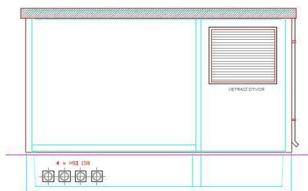
Pohľad C
