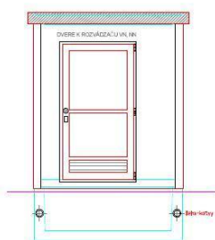
Pohľad B
