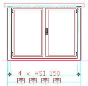
Pohľad A
