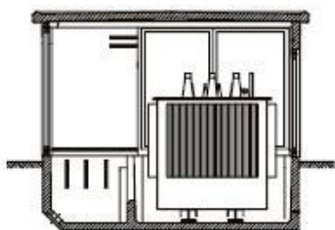
Pozdížny rez A.-A.
