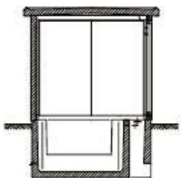
Priečny rez B.-B.
