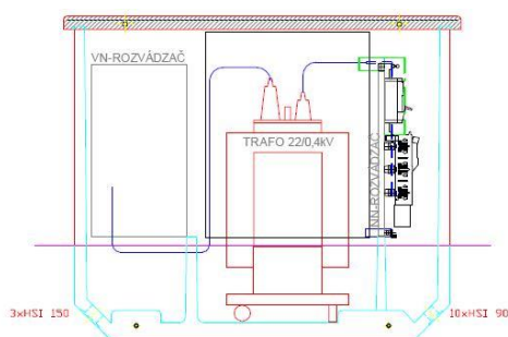
Priečny rez B-B
