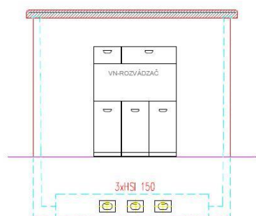
Priečny rez A-A
