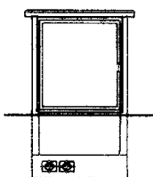
Pohled „B“ (strana VN rozvaděče)
