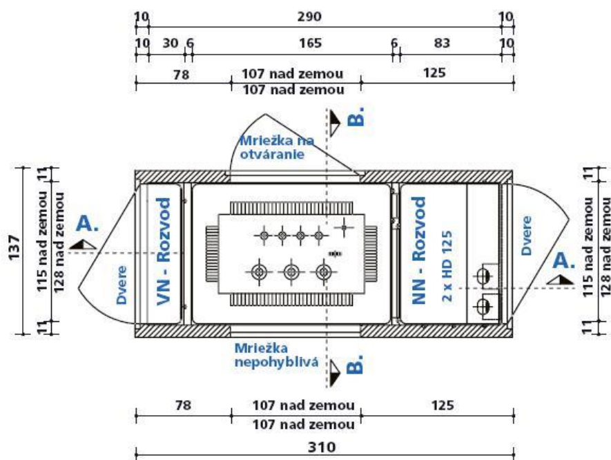
Situácia - pohľad zhora
