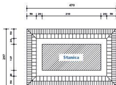
Situácia - pohľad zhora
