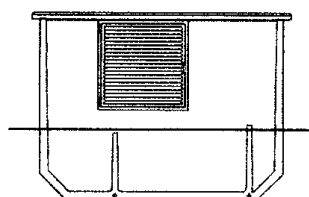
Ansicht „C“ (Seite TR)
